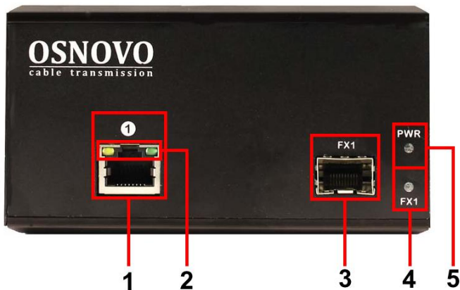
Рис. 2 Медиаконвертеры OMC-1000-11X/I, OMC-1000-11HX/I, разъемы, индикаторы, передняя панель
