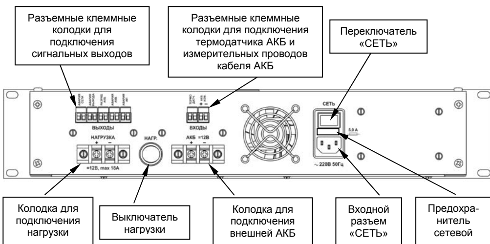
Рисунок 2 Общий вид задней панели источника
